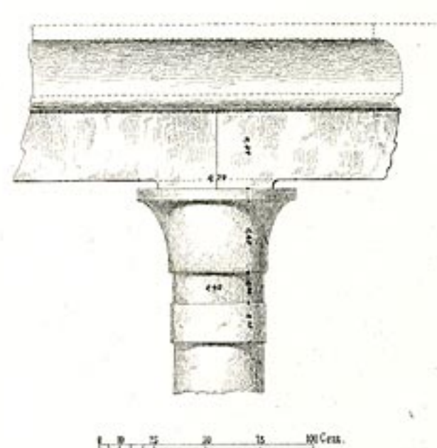
Säulenkapitäl.
